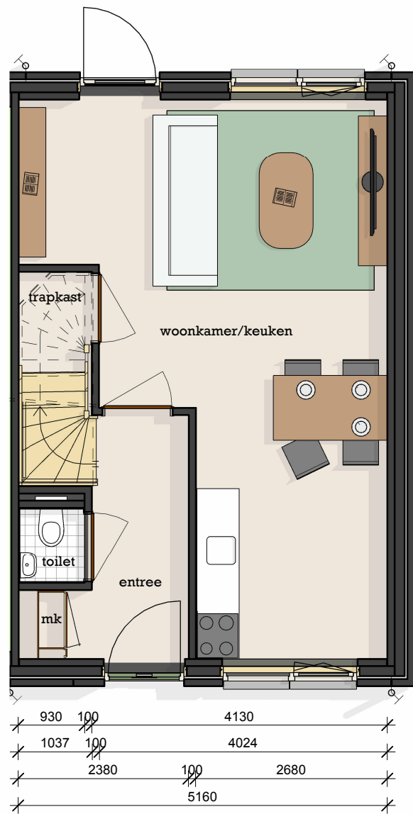
begane grond
